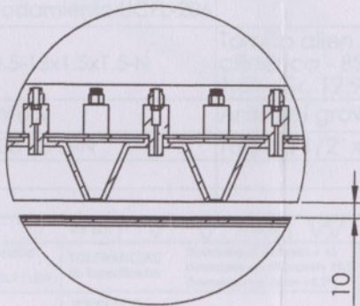
DETALLE A
