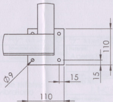
DETALLE B
