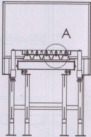
SECCION A-A
