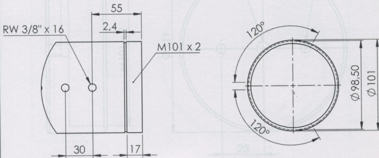
DETALLE B
