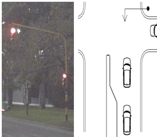
Figura 7 – Mal posicionamiento de unidades ópticas en un semáforo “vertical”
