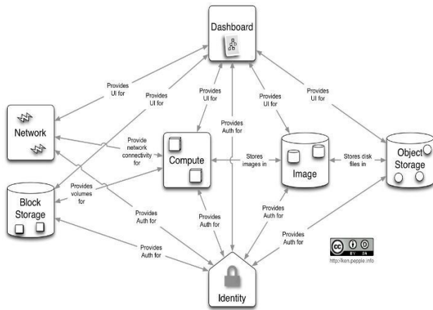
Fig. 1. Imagen representativa de la interconexión de módulos en OpenStack [7].
