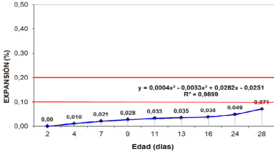
Figura 5 - Norma IRAM 1674 – Agregado Gravas del Rio Uruguay
