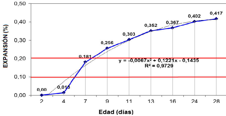
Figura 4 - Norma IRAM 1674 – Agregado Basáltico
