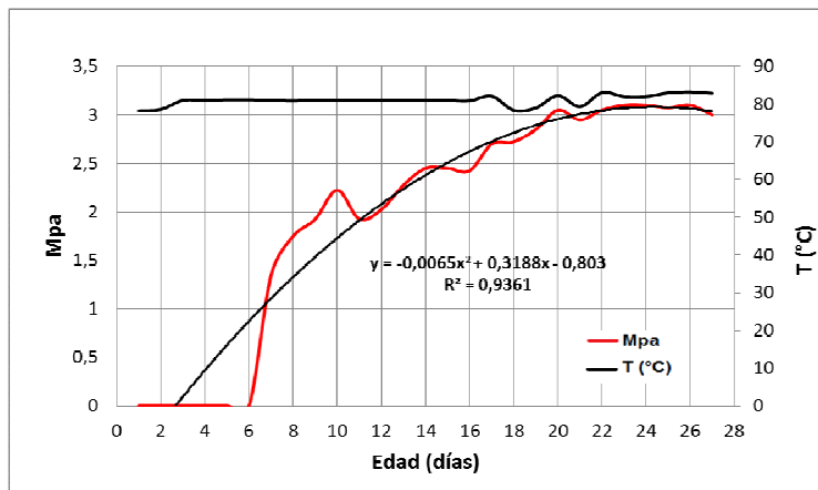
Figura 6 - Método de prueba PGAS – Agregado Basáltico
