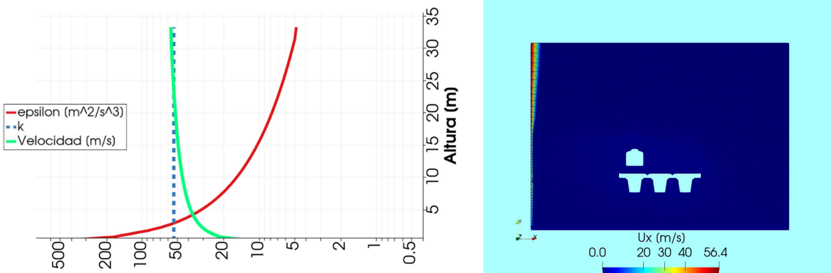
Figura 7: Distribución de velocidad, \kappa y \varepsilon en función de la altura implementada en el modelo como condición de contorno.
