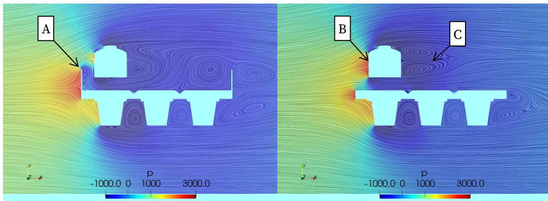
Figura 12: Campo de presiones y líneas de corriente para ambos casos evaluados.
