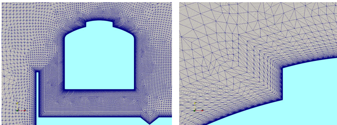
Figura 9: Detalle de la malla para el modelo con paneles final.
