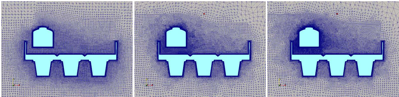
Figura 8: Mallas correspondientes al análisis de sensibilidad de malla para el caso con paneles.
