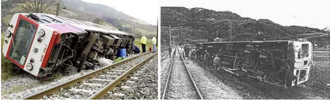
Figura 3: Vuelcos de trenes debido a la incidencia de viento cruzado: Austria (2002) -izq.- y Francia (1994) -der.- [3].
