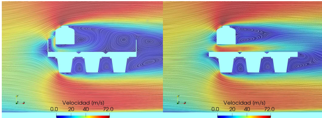
Figura 11: Campo de velocidades y líneas de corriente para ambos casos evaluados.
