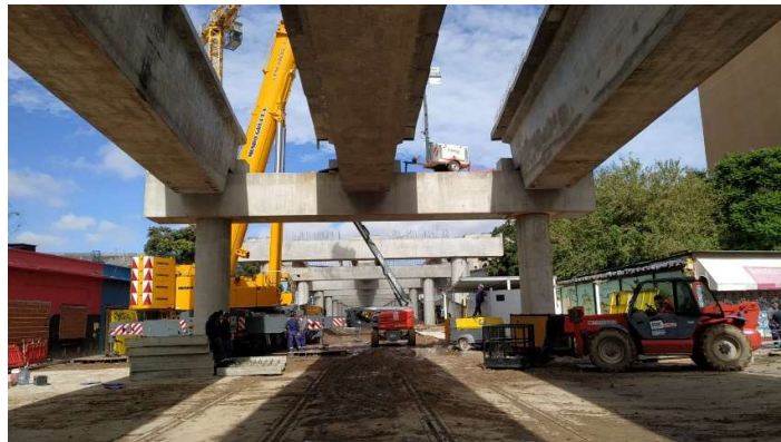
Figura 2: Construcción del viaducto
