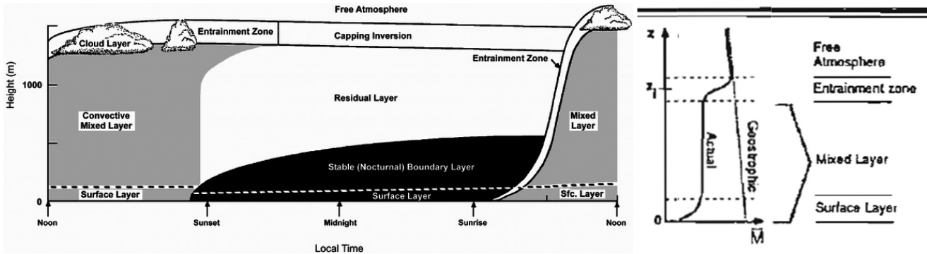
Figura 5: Capa límite terrestre y de superficie (izq.). Perfil de velocidad (M) típico para horario diurno (derecha). [9]
