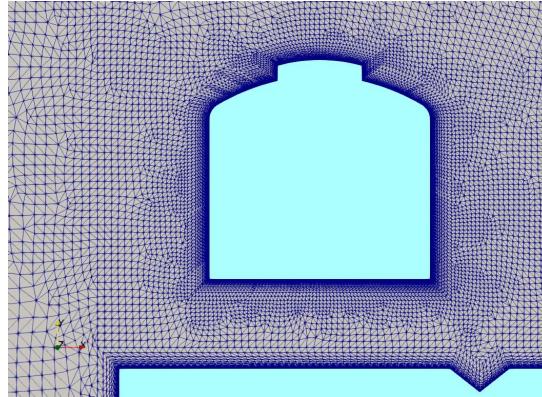
Figura 10: Detalle de la malla para el modelo sin paneles final.
