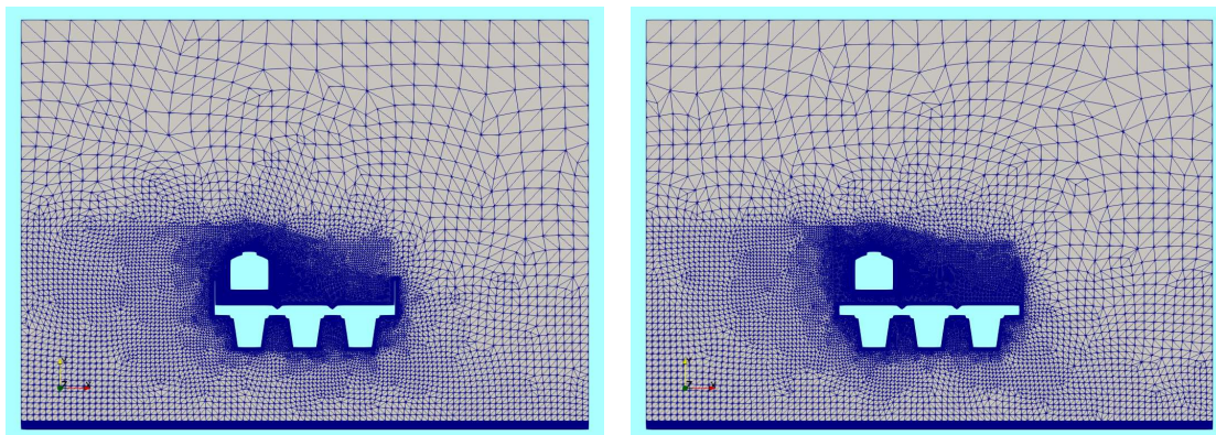
Figura 6: Malla del modelo numérico implementado para el caso con paneles (izq.) y sin paneles (der.).
