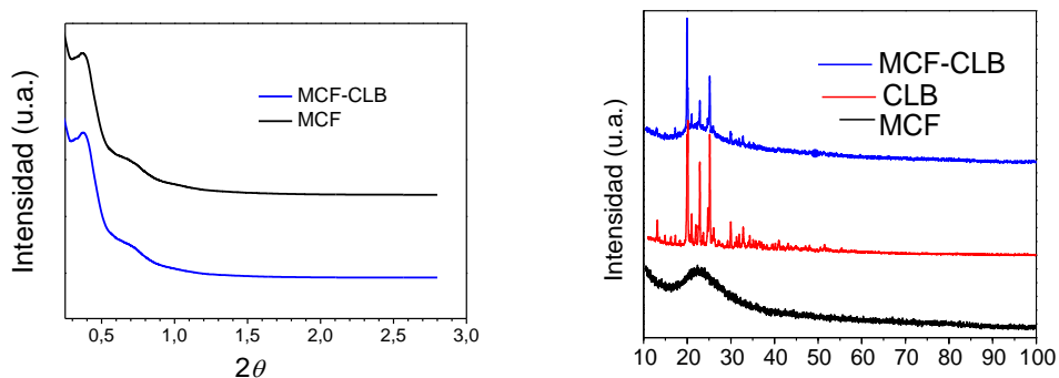
Figura 1: Patrón de Rayos X del hospedaje y del composite.
